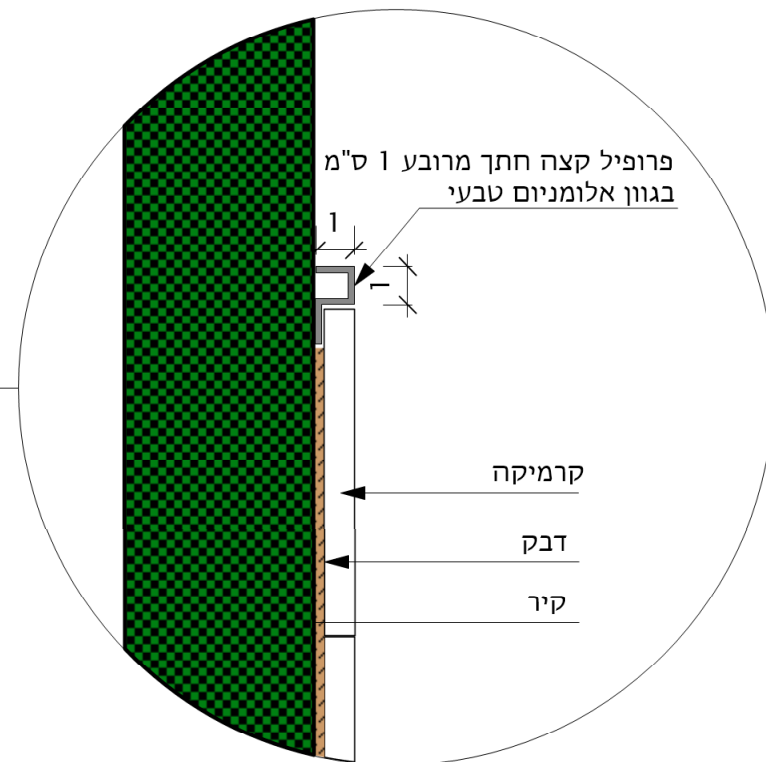
פרט פרופיל קצה / פינה
