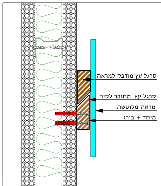
פרט תליית מראה
