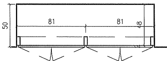
תוכנית 1:25
