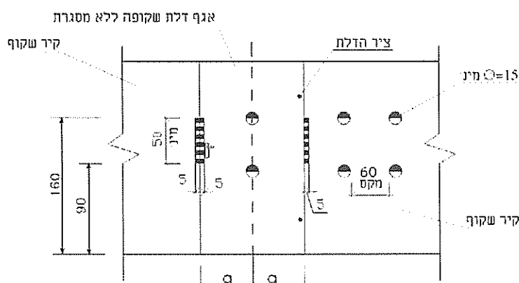
12ג - סימון דלת שקופה משולבת בקיר שקוף
