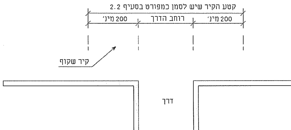
12א - סימון קירות שקופים – מבט על
