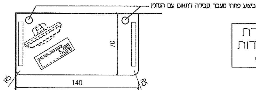
תוכנית 1:25
