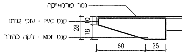
פרט קצה שולחן - בכל קצה כתוח
