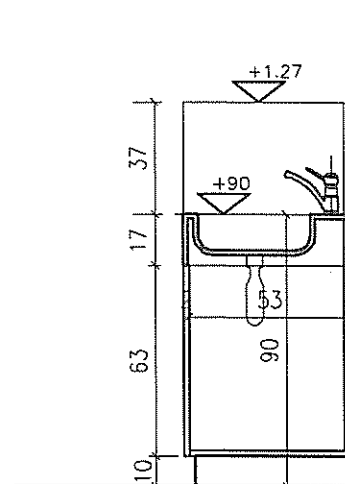
חתך 1:25
