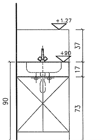
חזית 1:25
