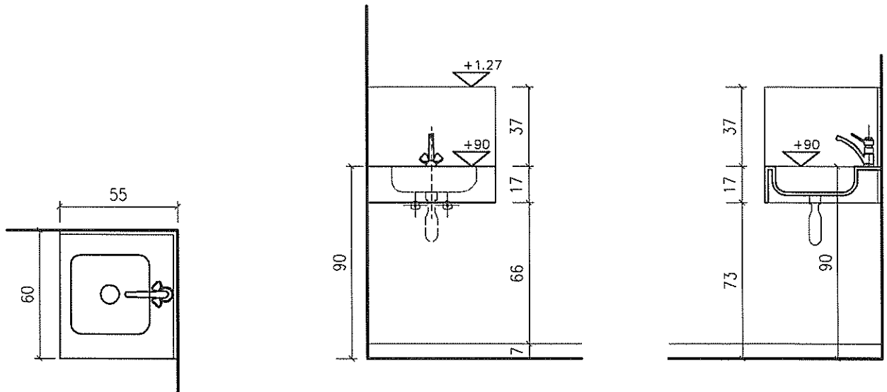
תוכנית 1:25
