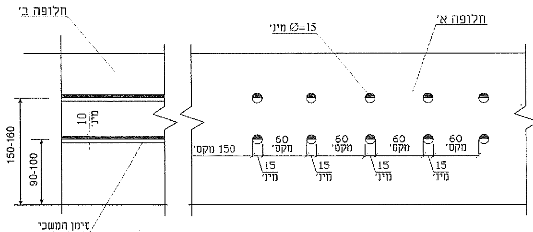
12ב - סימון קירות שקופים – חזית
