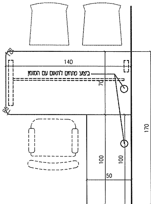
תוכנית 1:25
