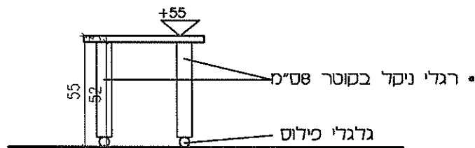
חתך 1:25
