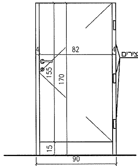
חזית 1:25
