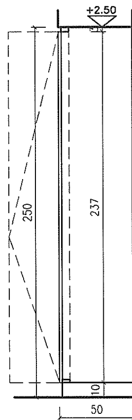
חתך 1:25
