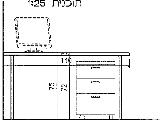
תוכנית 1:25
