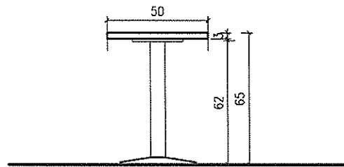
חתך 1:25
