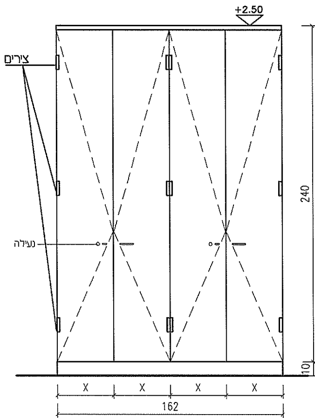
חזית 1:25
