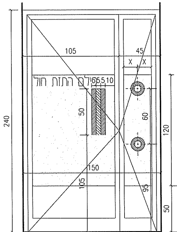
חזית 1:25
