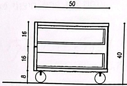
חתך אנכי א'-א'
